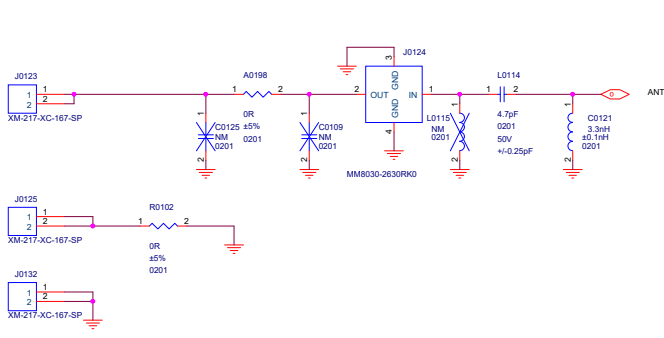
ANT12_N78_79_DRXM
