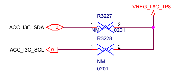
ACC
