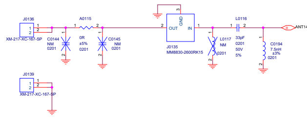
ANT14
