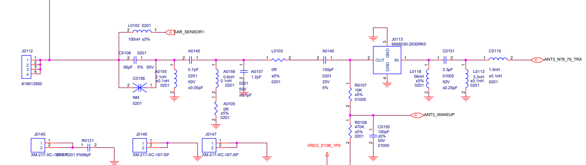
ANT3_N78_79_TRX
