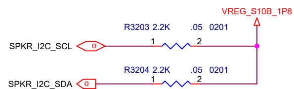
ADSP I2C
