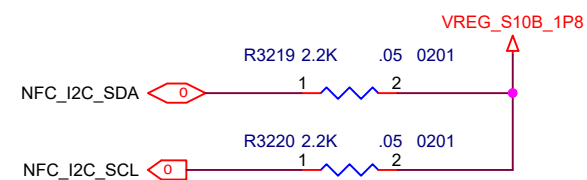
NFC I2C
